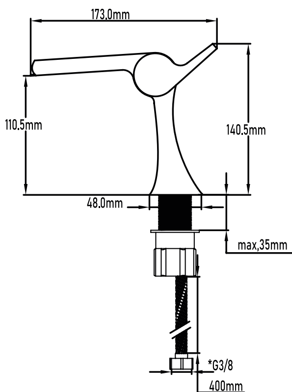
PLANO TÉCNICO
